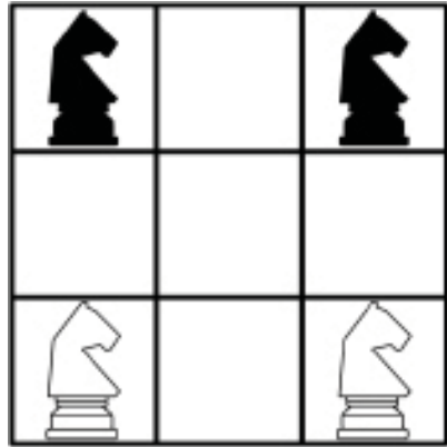
Afbeelding 1. Het probleem van Guarini: verwissel de paarden
