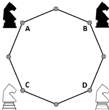
Afbeelding 2: Het schaakbord negeren en het diagram uitvouwen
