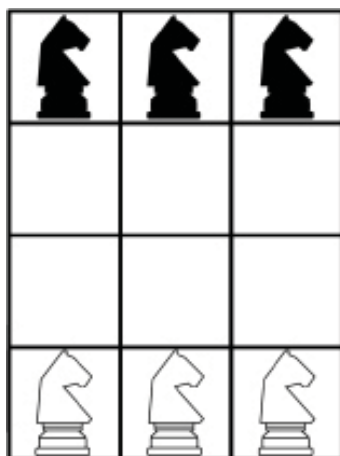
Afbeelding 3: Verwissel de paarden
